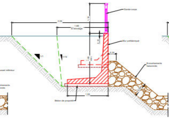
COUPE C-C (Scale 1/200)
