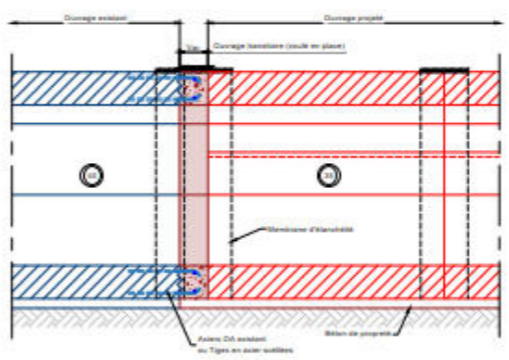
COUPE SUR OUVRAGE DE TRANSITION (Scale 1/200)
