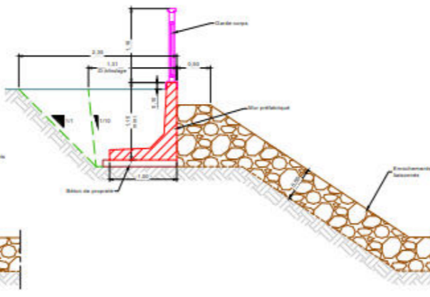
COUPE D-D (Scale 1/200)
